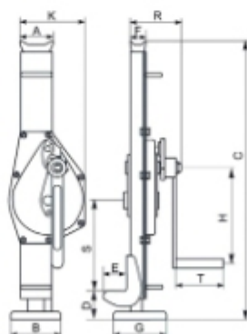
Рисунок 1. Размеры домкрата.
